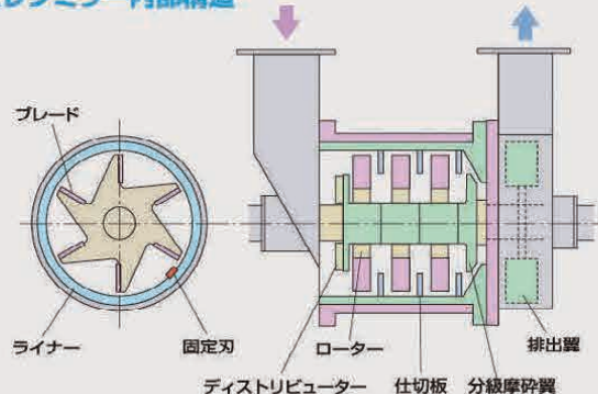
セレンミラー内部構造
